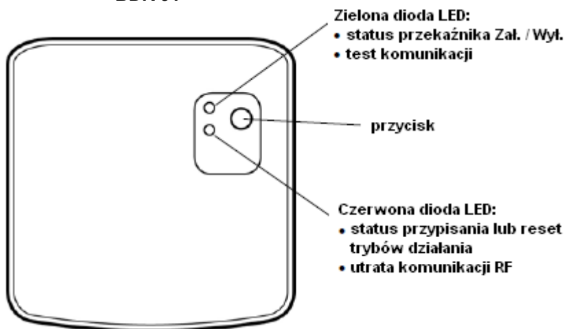
Skrzynka przekaźnikowa BDR 91
