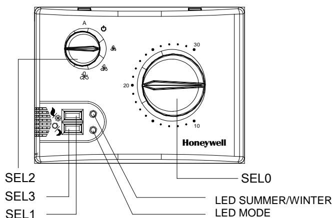
Rys. 9 Ustawianie parametrów (dotyczy tylko T6580A1008)
