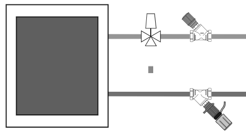
Rys. 7. Kombi-3-plus z siłownikiem termicznym w nagrzewnicy / klimakonwektorze
