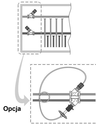
Rys. 6. Kombi-3-plus na rozdzielaczu
