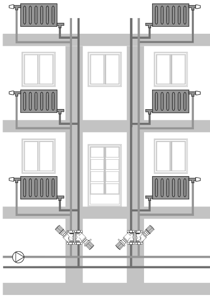
Rys. 4. Kombi-3-plus CZERWONY i NIEBIESKI w pionach
